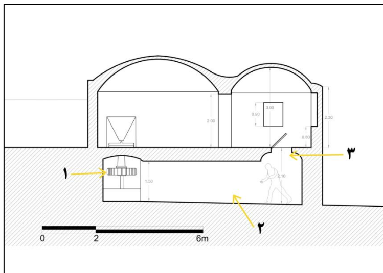
شکل ۱۶: برش A-A (۱) پره (۲) چدی (۳) چاه چیه
